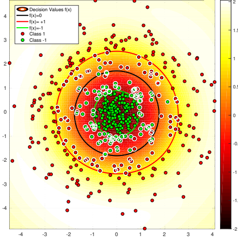
(a) \nu=0.32, \sigma=2.014, \text{SV}=164, \text{ACC}=0.97
